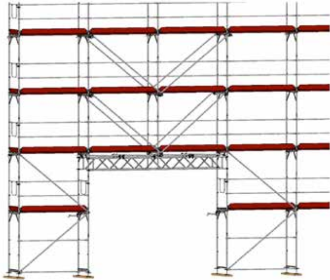
Bild 54: Überbrückung
