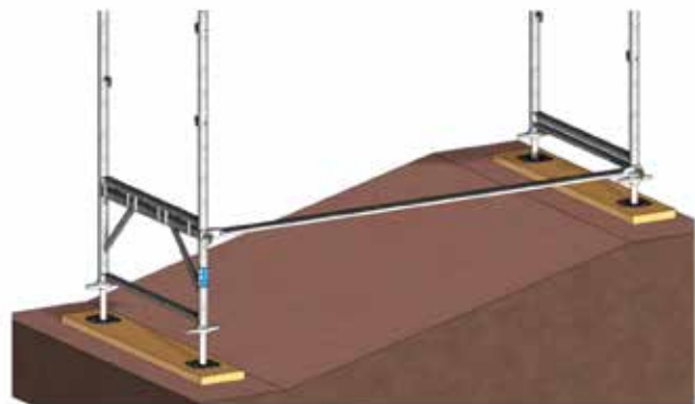
Bild 5: Ausgleichsrahmen mit 0,50 m bzw. 1,00 m Höhe.
