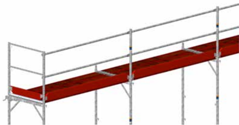
Bild 46: Vollständiger Seitenschutz
