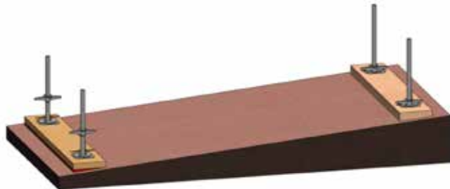
Bild 2: Lastverteiler Unterbau auf geneigter Fläche
