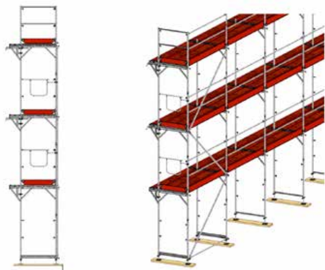
Bild 50: Gerüst mit Verbreiterungskonsolen innen
