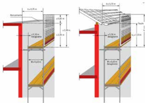
Bild 59: Schutzwand mit Maßangaben
