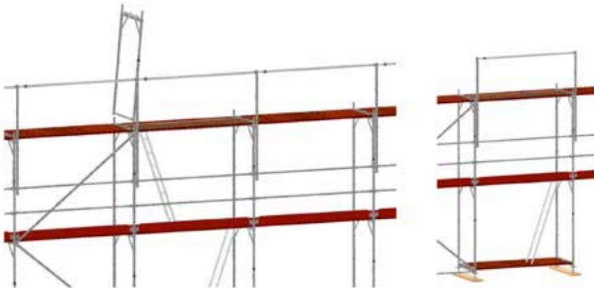
Bild 31: Aufstecken eines Vertikalrahmens.
